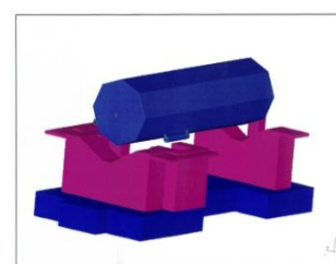
Massif broyeur : étude dynamique
