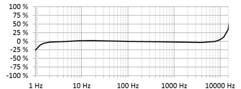
Courbe de réponse du Dygit1®
